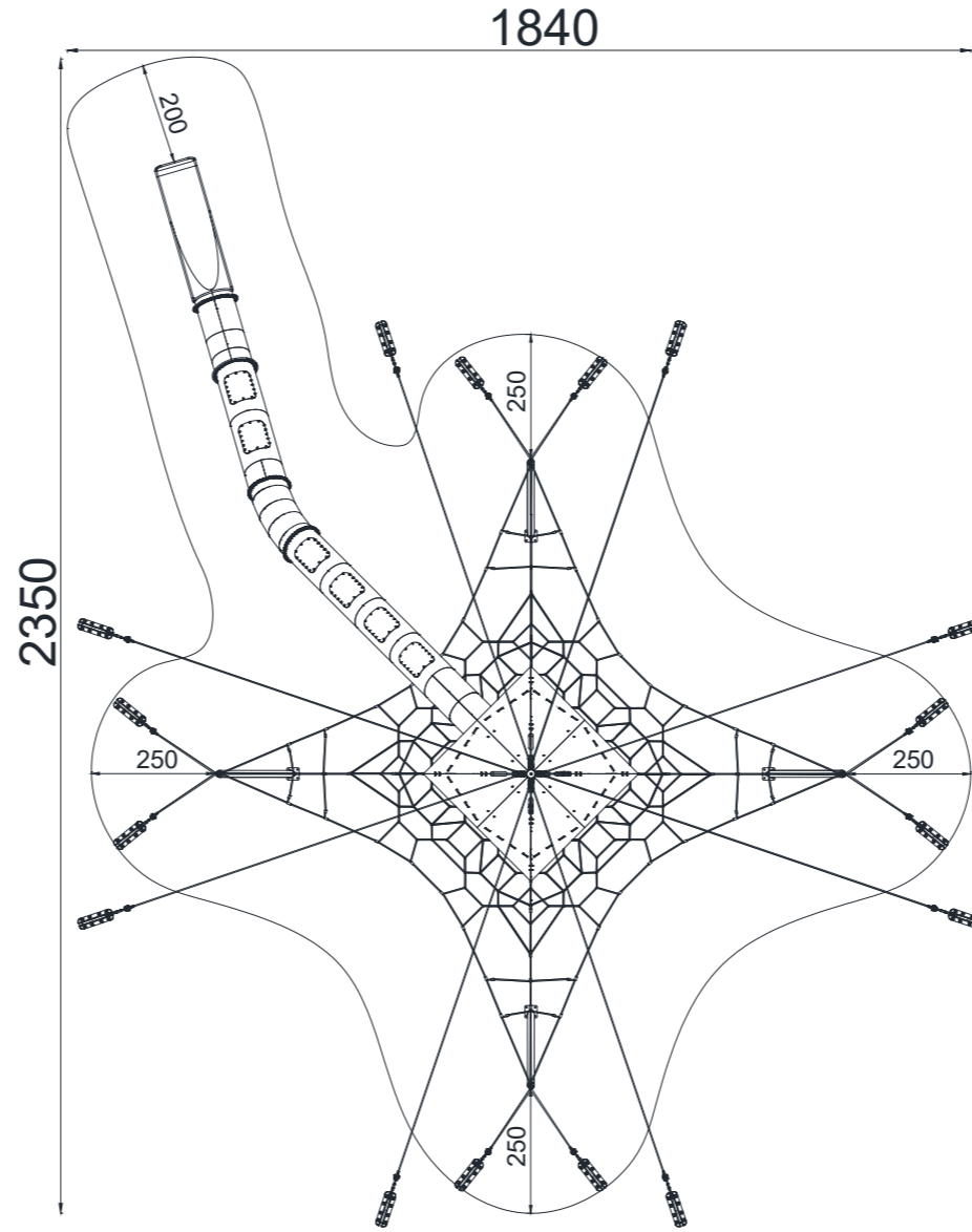
ÜST GÖRÜNÜŞ / TOP VIEW
