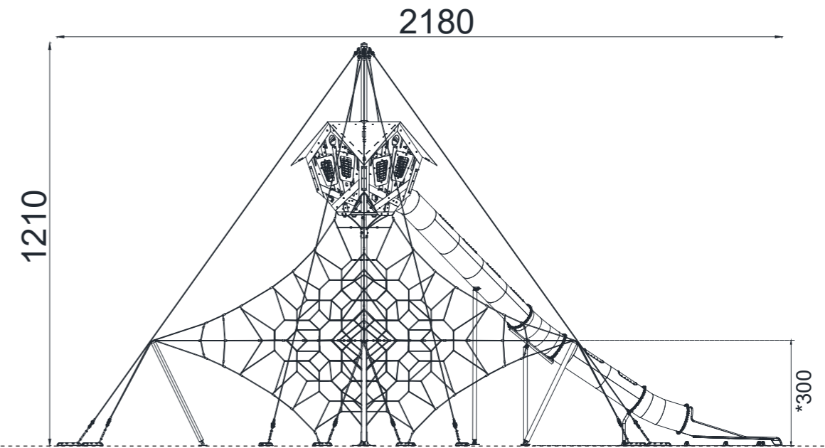
YAN GÖRÜNÜŞ / SIDE VIEW
