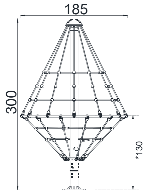
ÖN GÖRÜNÜŞ / FRONT VIEW
