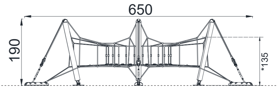
YAN GÖRÜNÜŞ / SIDE VIEW
