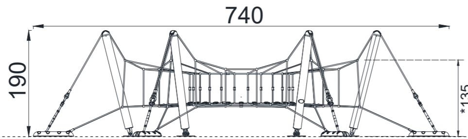
ÖN GÖRÜNÜŞ / FRONT VIEW
