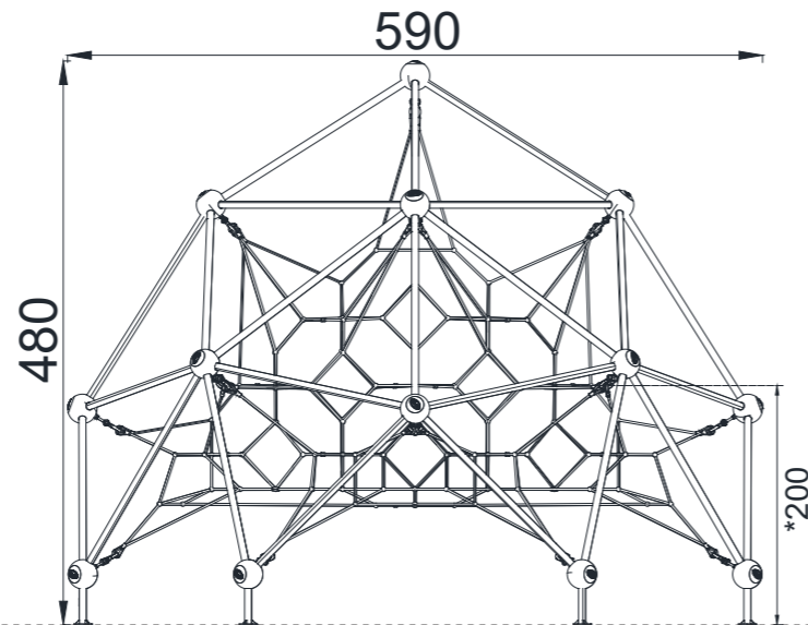
ÖN GÖRÜNÜŞ / FRONT VIEW
