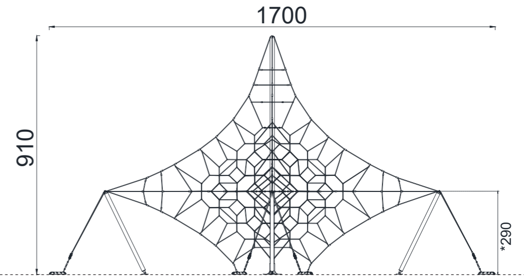
YAN GÖRÜNÜŞ / SIDE VIEW
