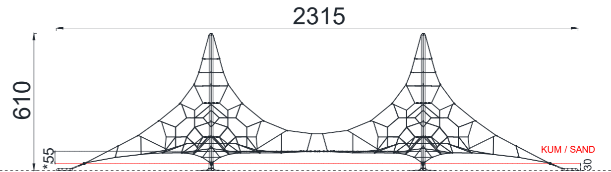
YAN GÖRÜNÜŞ / SIDE VIEW
