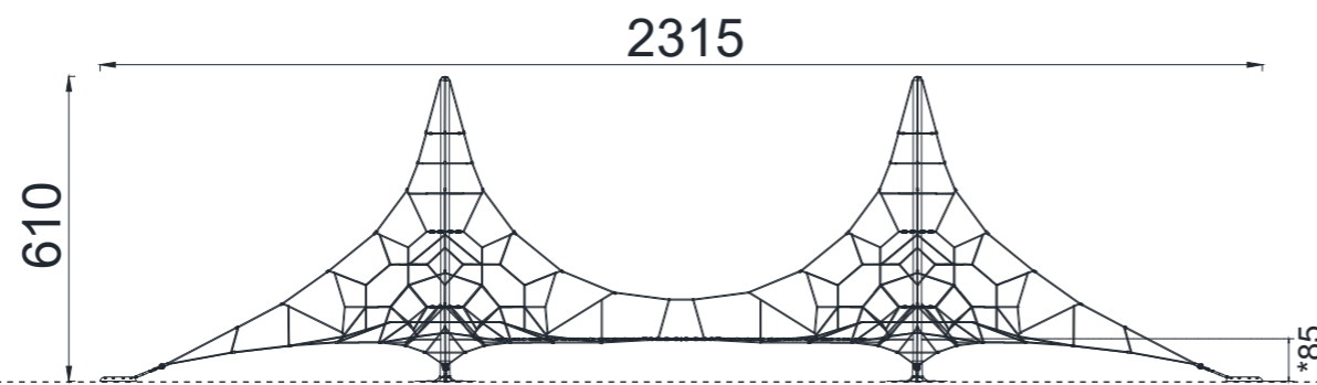
ÖN GÖRÜNÜŞ / FRONT VIEW
