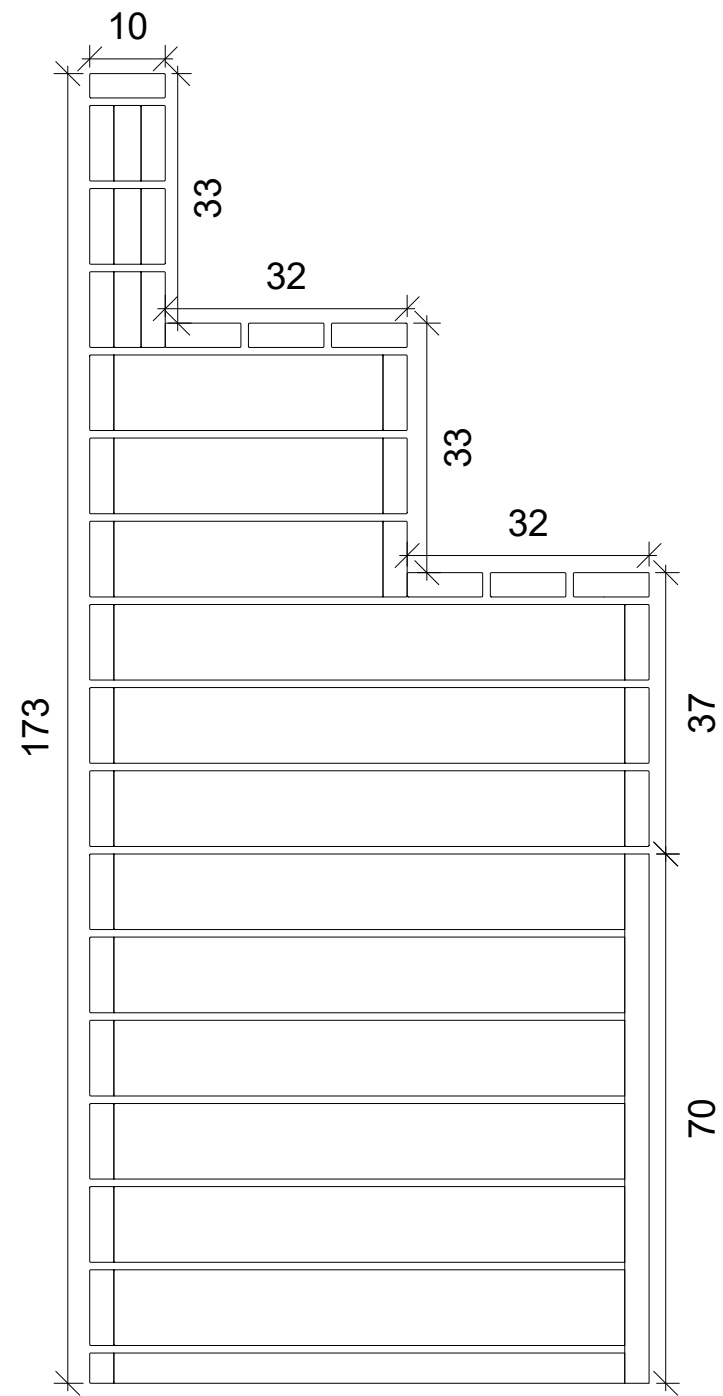
① Opstalt 1 : 10
